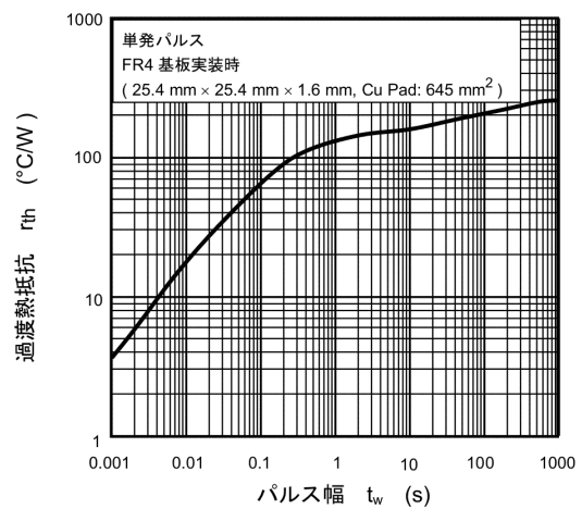
図 7.12 r th - t w
