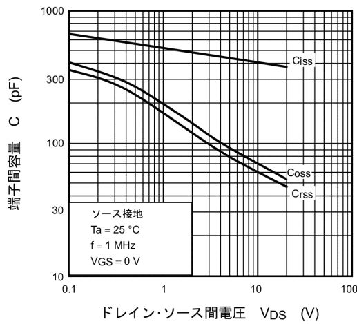
図 7.9 C - V DS
