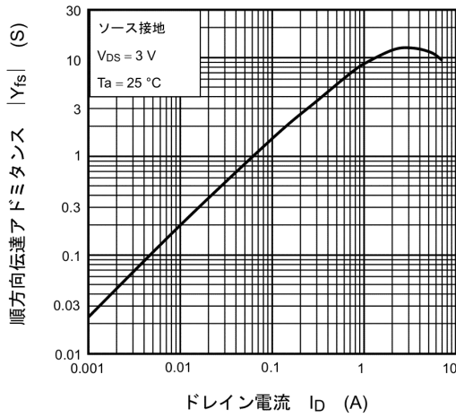
図 7.7 |Y fs | - I D
