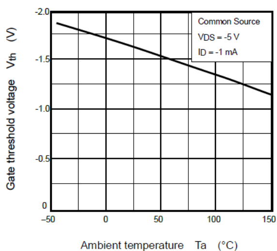
Fig. 7.6 V_{th} - T_a
