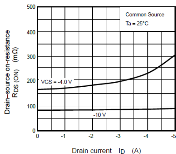
Fig. 7.4 R_{DS(ON)} - I_D
