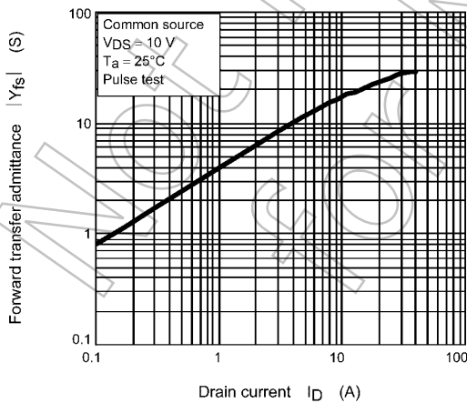
Fig. 8.5 |Y_{fs}| - I_D
