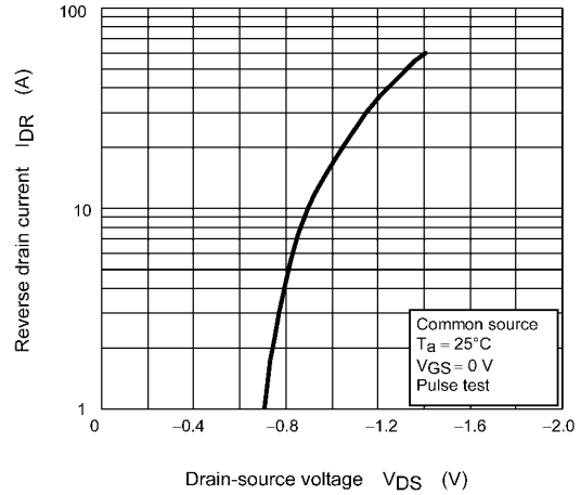
Fig. 8.8 I_{DR} - V_{DS}
