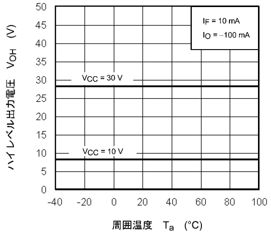
図 12.2.8 V_{OH} - T_a
