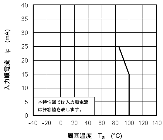
図 12.2.2 I_F - T_a
