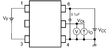
図 12.1.2 I OPL 測定回路
