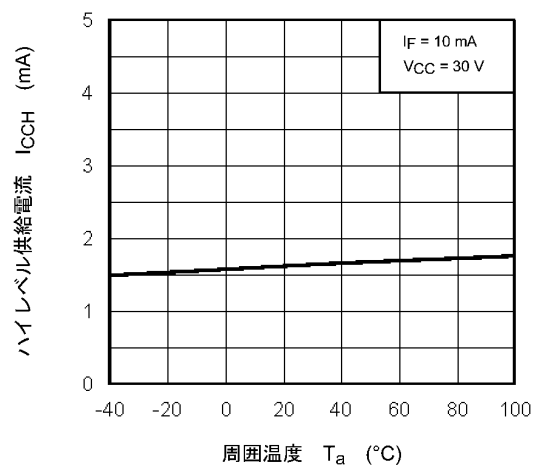
図 12.2.6 I_{CCH} - T_a
