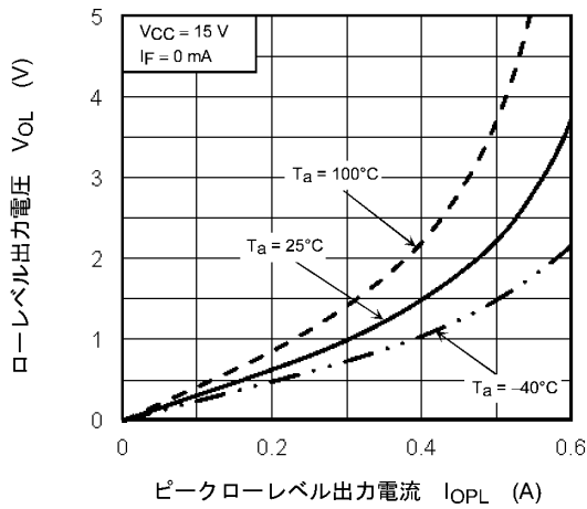
図 12.2.9 V_{OL} - I_{OPL}
