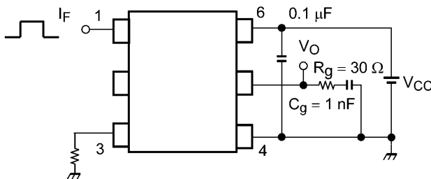
図 12.1.7 伝搬遅延時間測定回路, 波形
