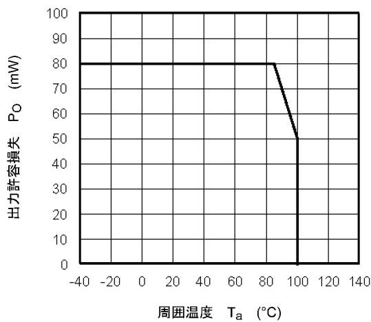
図 12.2.3 P_O - T_a
