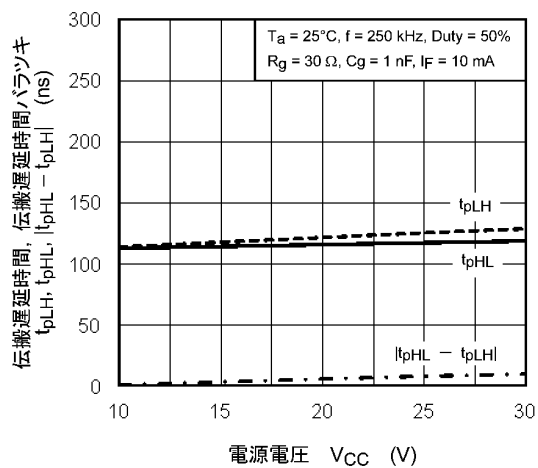
図 12.2.13 t_{pLH}, t_{pHL}, |t_{pHL} - t_{pLH}| - V_{CC}
