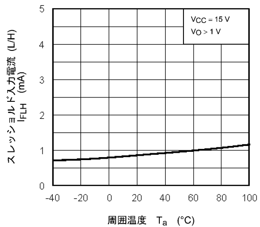
図 12.2.4 I_{FLH} - T_a
