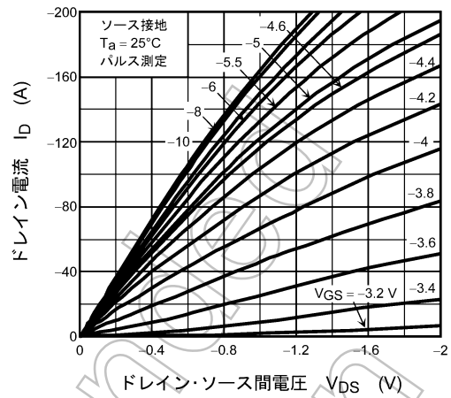
図 9.2 I_D - V_{DS}
