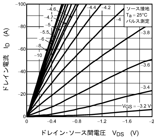
図 9.1 I_D - V_{DS}
