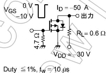
図 6.2.1 スwitching時間の測定回路
