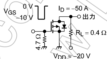
図 6.2.1 スwitching時間の測定回路
