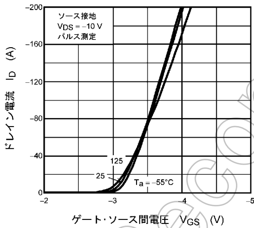
図 9.3 I_D - V_{GS}
