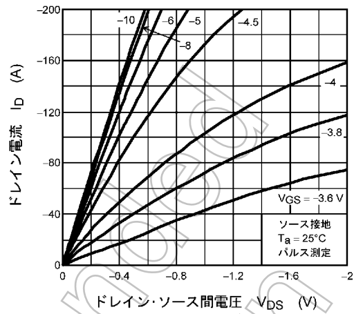
図 9.2 I_D - V_{DS}
