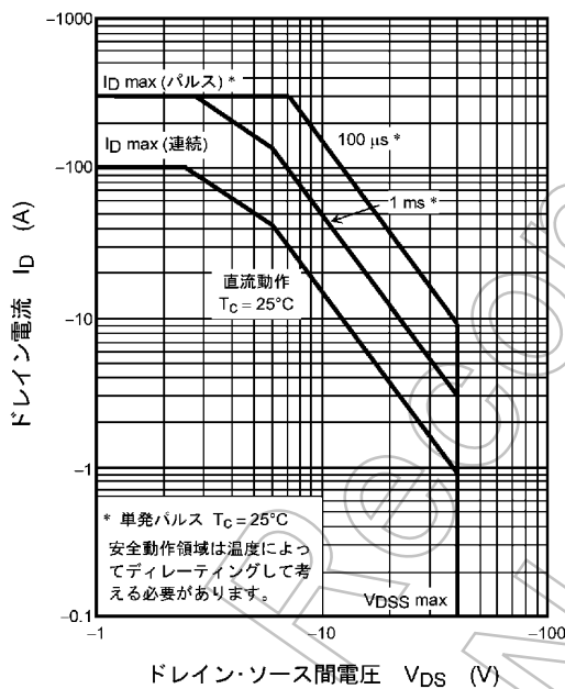
図 9.13 安全動作領域 (最大値 (保証値))
