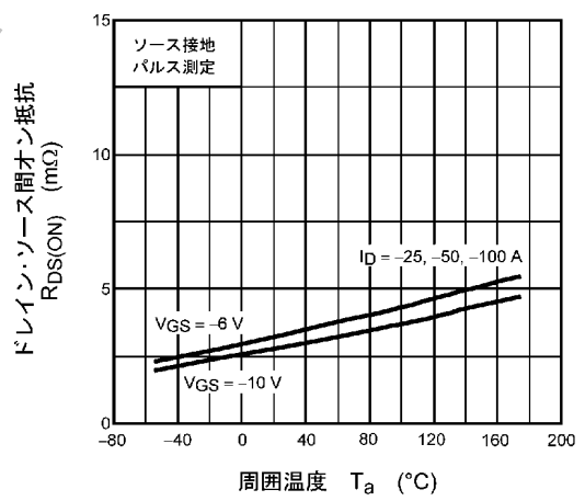
図 9.6 R_{DS(ON)} - T_a
