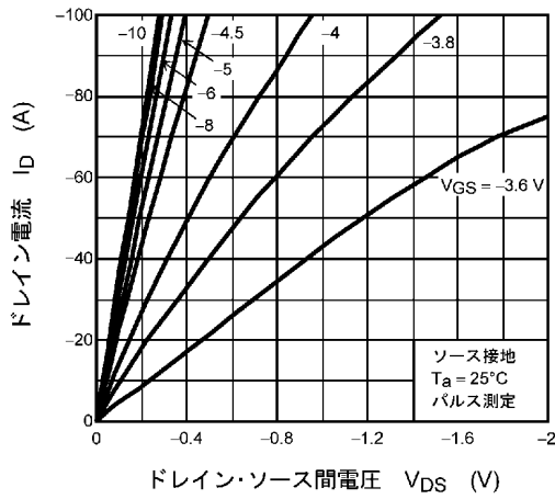
図 9.1 I_D - V_{DS}
