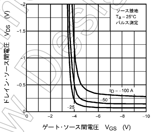
図 9.4 V_{DS} - V_{GS}
