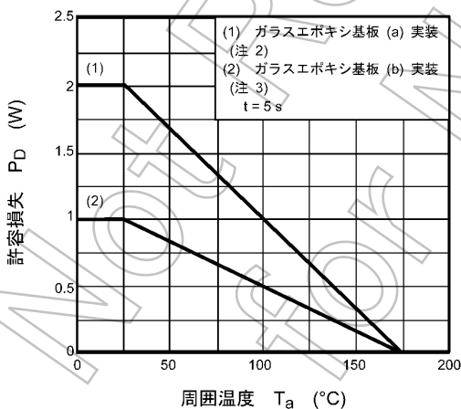
図 8.11 P_D - T_a (最大値 (保証値)) (注8)
