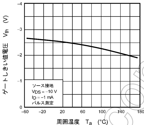
図 8.9 V_{th} - T_a (注8)
