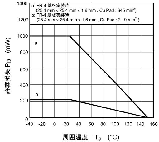
図 7.14 P_D - T_a
