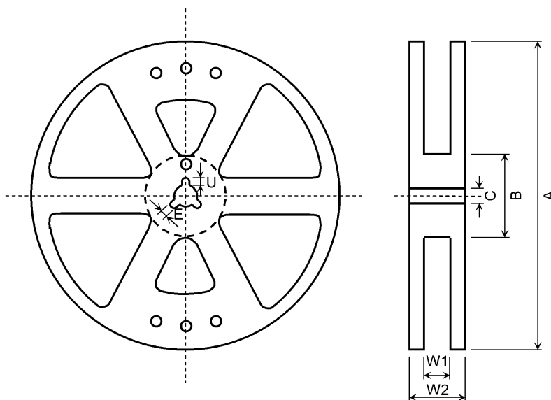
図 16.3.6.1 リール形状
