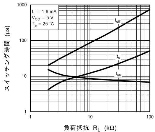
図 11.16 スwitching時間 - R_L
