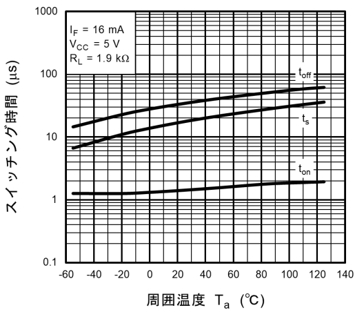
図 11.15 スwitching時間 - T_a
