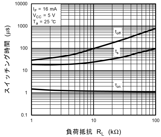
図 11.14 スwitching時間 - R_L
