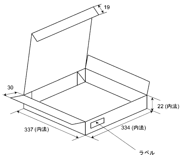
1リール入り梱包箱 (unit: mm)
