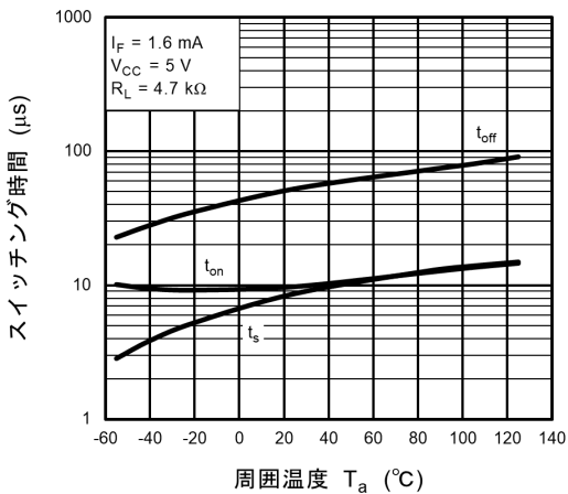
図 11.17 スwitching時間 - T_a
