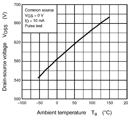
Fig. 8.5 V_{DSS} - T_a
