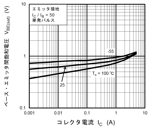
図 7.4 V_{BE(sat)} - I_C
