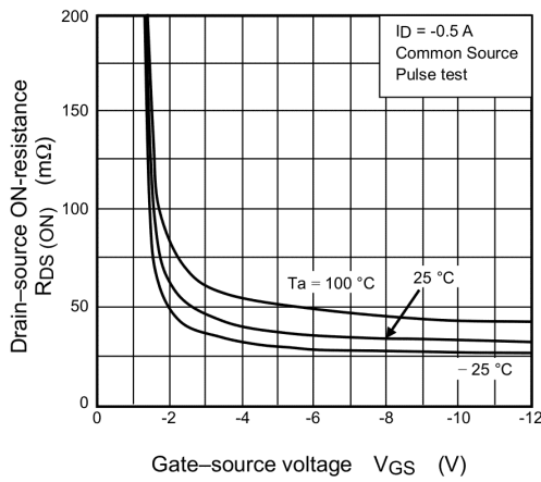
Fig. 8.3 R_{DS(ON)} - V_{GS}
