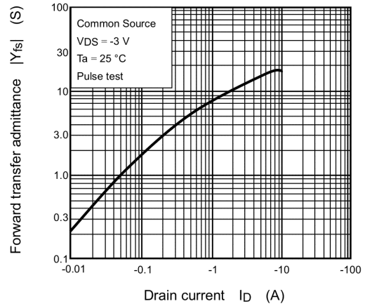
Fig. 8.8 |Y_{fs}| - I_D
