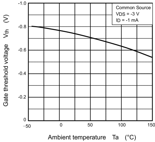
Fig. 8.7 V_{th} - T_a
