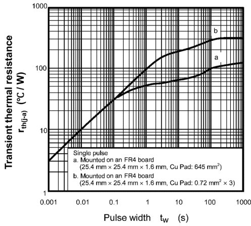
Fig. 8.13 r_{th(j-a)} - t_w
