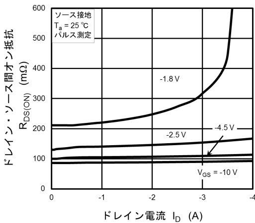
図 7.5 R_{DS(ON)} - I_D
