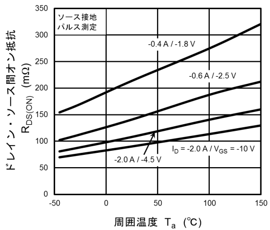
図 7.6 R_{DS(ON)} - T_a
