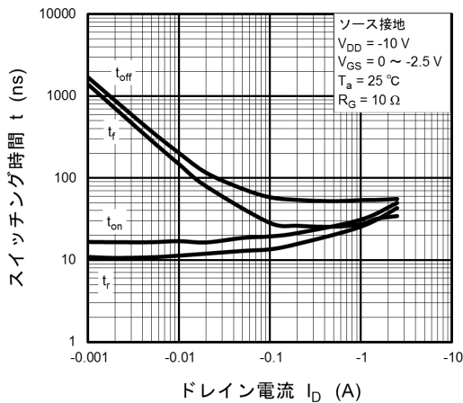
図 7.11 t - I_D
