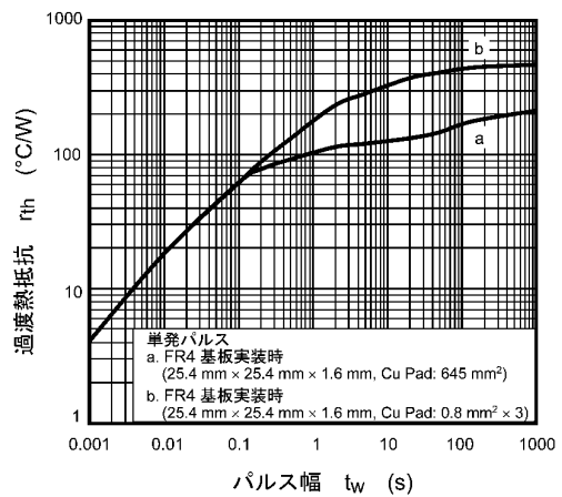
図 7.12 r_{th} - t_w
