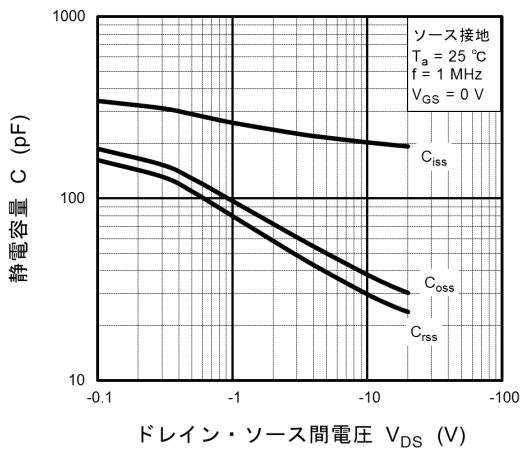
図 7.9 C - V_{DS}
