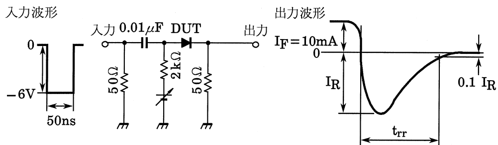
図1. 逆回復時間 ( t_{rr} ) 測定回路
