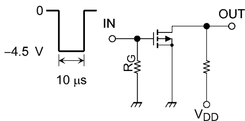
図 5.3.1 スwitchング時間の測定回路
