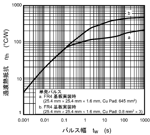
図 7.11 r_{th} - t_w
