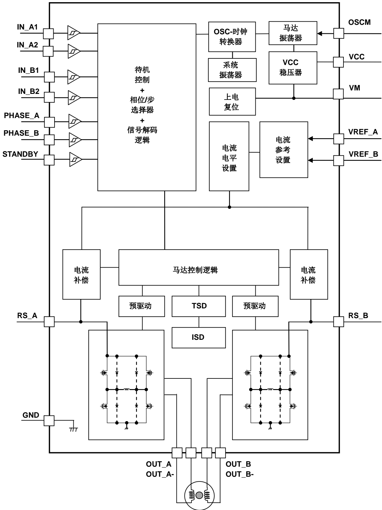
TB62261FTAG 方块图
