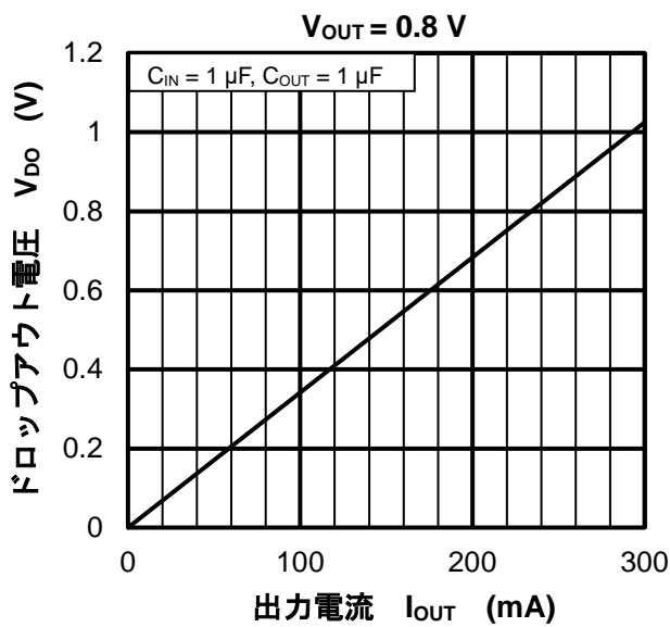
ドロップアウト電圧—出力電流特性
