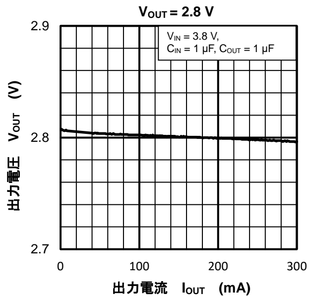
出力電圧—出力電流特性
