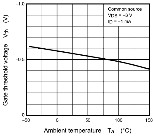
Fig. 7.7 V_{th} - T_a
