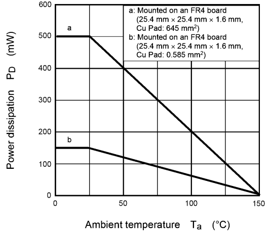
Fig. 7.14 P_D - T_a
