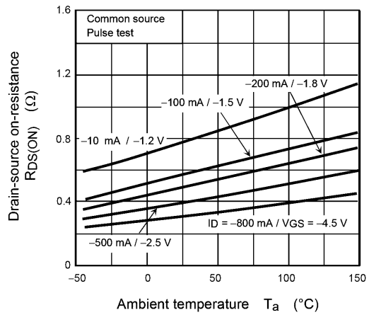
Fig. 7.6 R_{DS(ON)} - T_a
