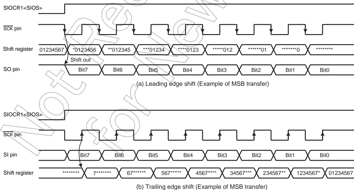
Figure 10-4 Shift Edge
