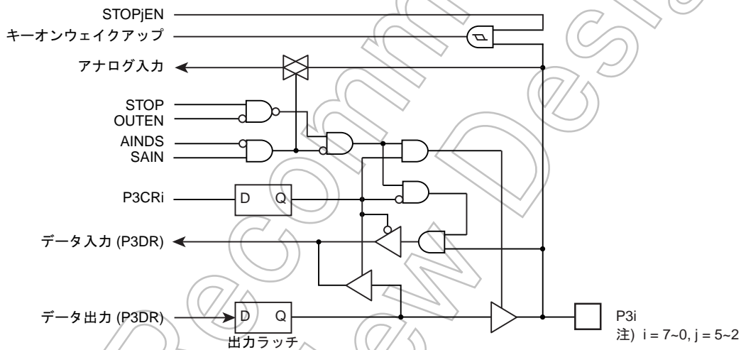
図 7-5 P3 ポート
