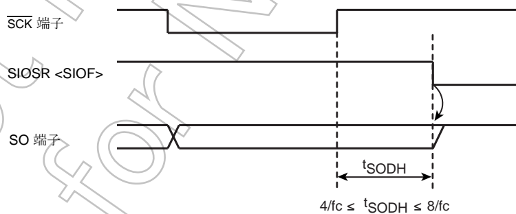
図 10-17 送受信終了時のデータ保持時間
