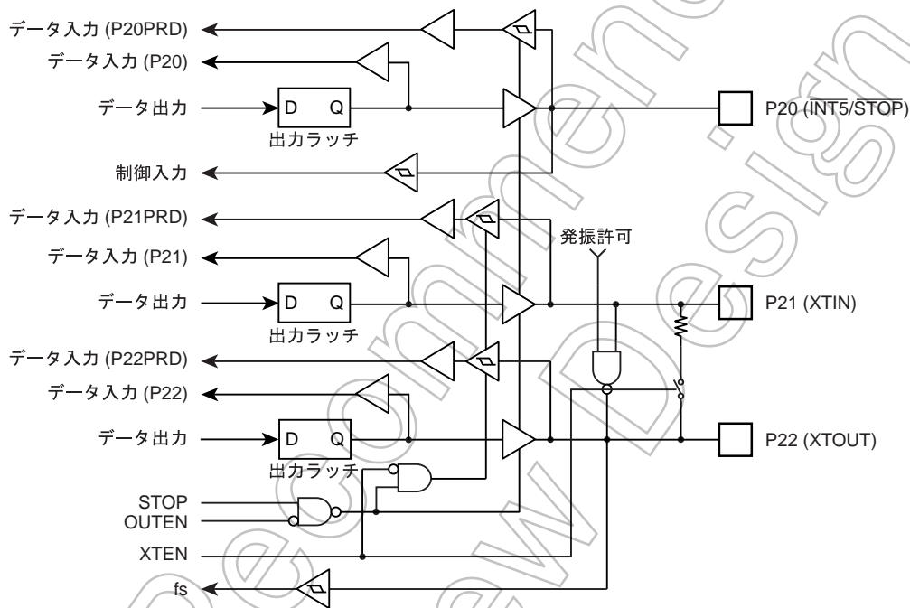
図 7-4 P2 ポート
