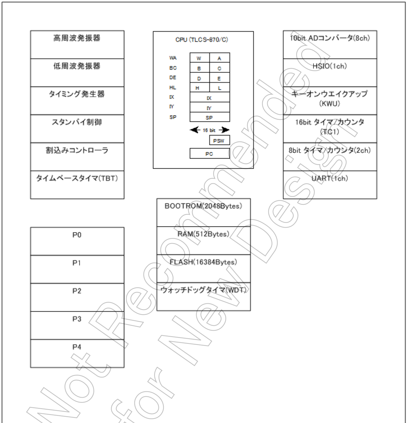
図 1-2 ブロック図
