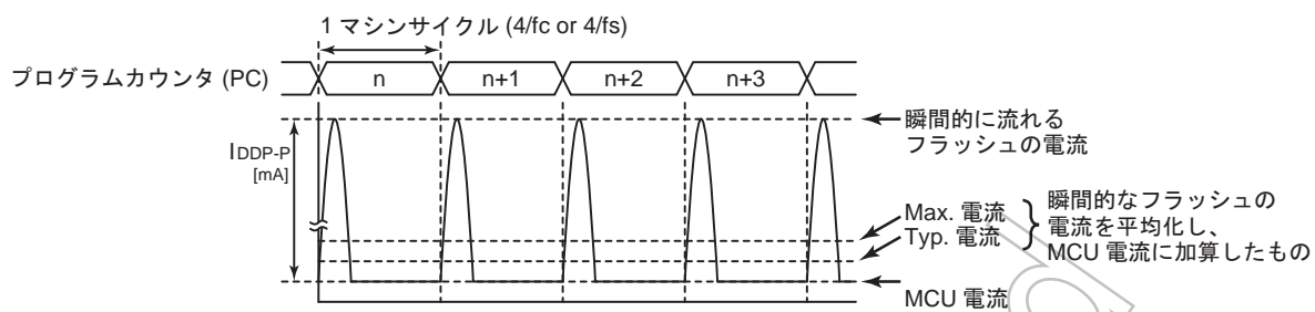
図 17-1 フラッシュメモリの間欠動作
