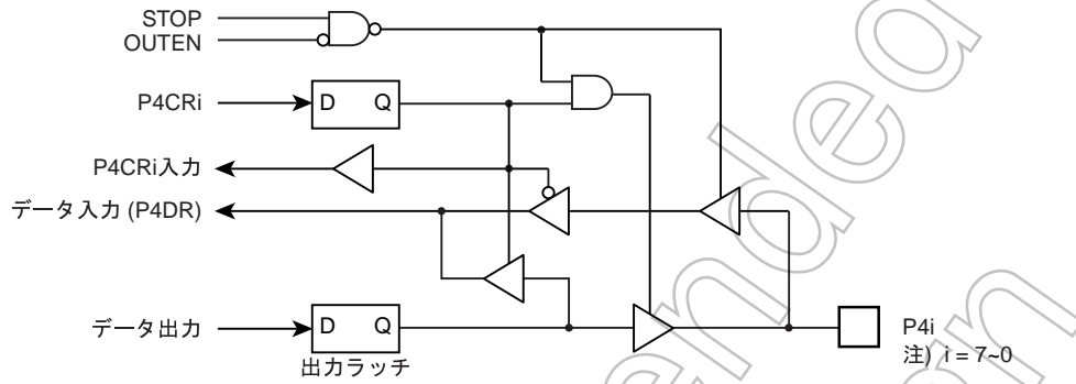
図 7-6 P4 ポート
