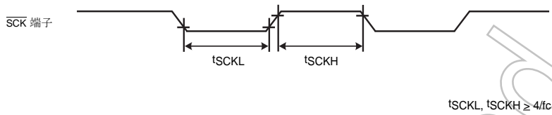
図 10-3 外部クロック
