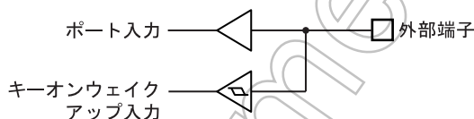
図 13-2 キーオンウェイクアップ入力とポート入力
