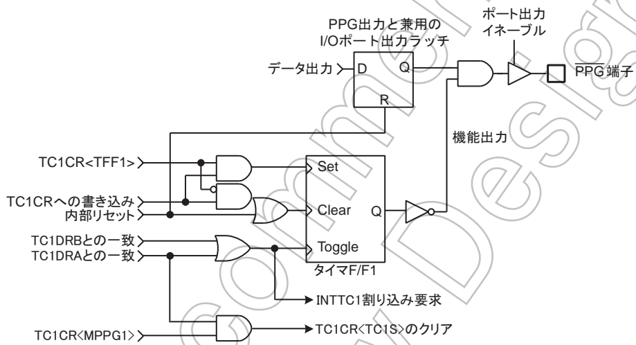
図 8-7 PPG 出力
