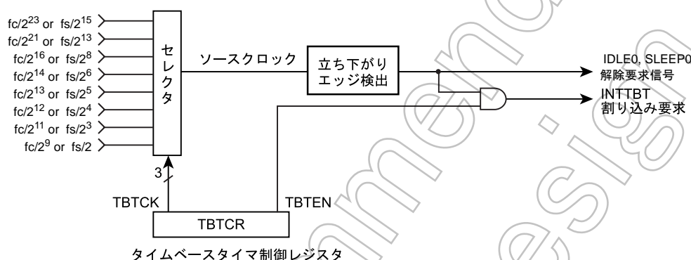
図 5-1 タイムベースタイマの構成
