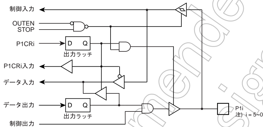
図 7-3 P1 ポート
