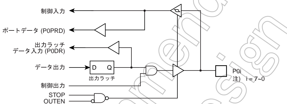
図 7-2 P0 ポート
