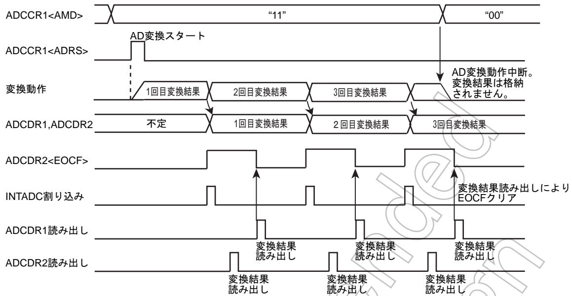
図 12-3 リpeatモード
