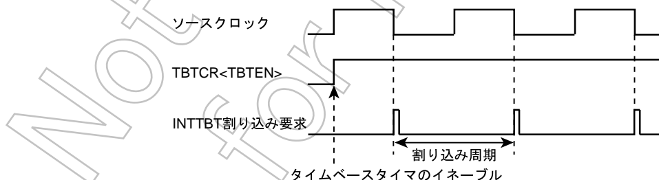
図 5-2 タイムベースタイマ割り込み
