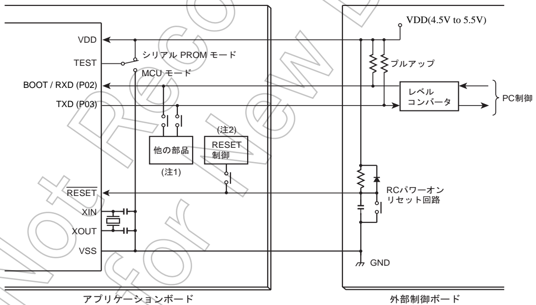
図 15-3 オンボード書き込み接続例
