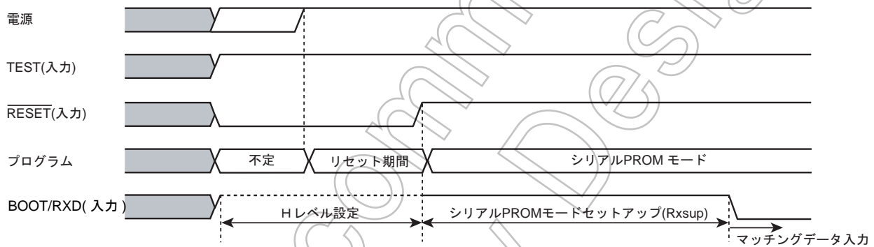
図 15-4 シリアル PROM モードタイミング
