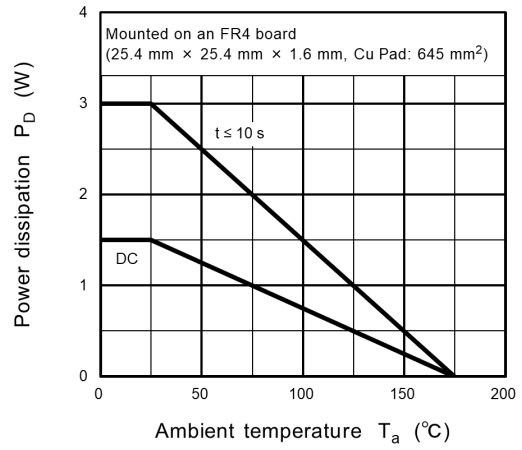
Fig. 7.14 P_D - T_a
