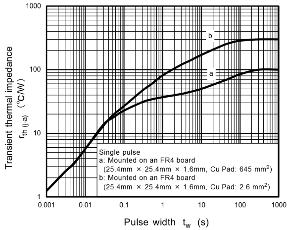
Fig. 7.13 r_{th} - t_w
