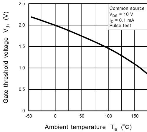
Fig. 7.7 V_{th} - T_a
