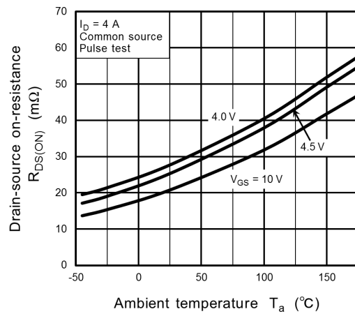
Fig. 7.6 R_{DS(ON)} - T_a
