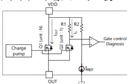
図 4.3 通電検出回路概略
