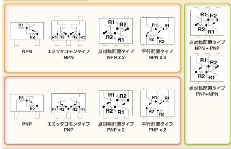
内部接続図
