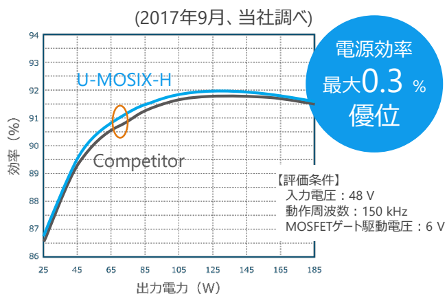
フルブリッジDC-DCコンバーターでの効率比較
