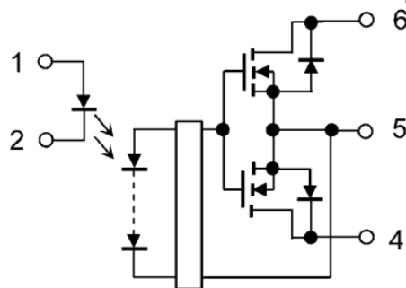
TLP3545A 内部等価回路
