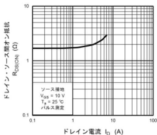
TK2K2A60F 特性図
