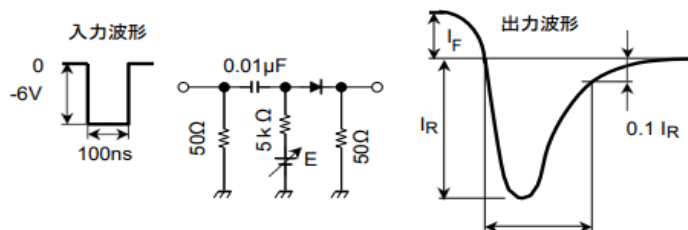
順電圧 と 逆電圧時の動作 \tau
