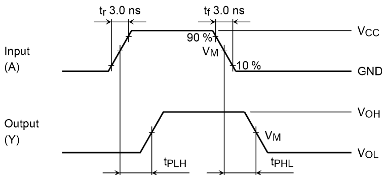
Fig. 9.8.1 t_{PLH} , t_{PHL}
