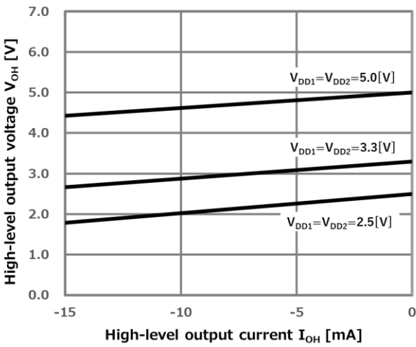
Fig.13.7. V_{OH}-I_{OH}
