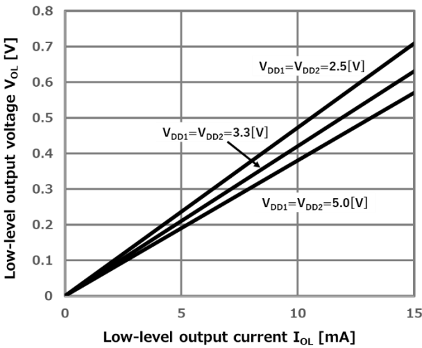
Fig.13.8. V_{OL}-I_{OL}
