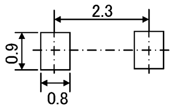
図 8.1 参考パッド寸法 (Unit: mm)
