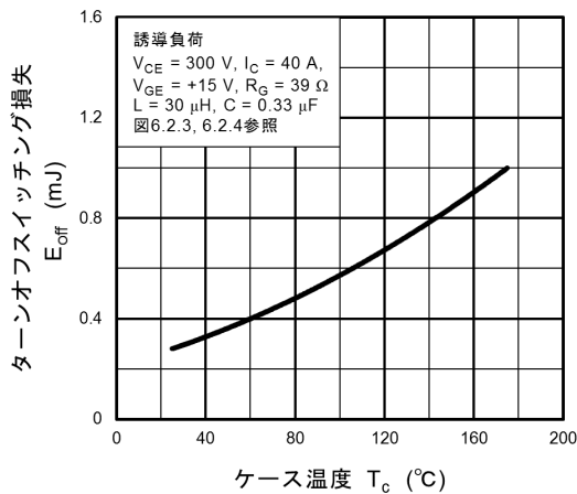
図 8.17 E_{\text{off}} - T_c
