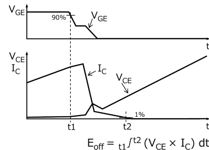
図 6.2.4 スwitchング損失のタイミングチャート
