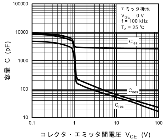
図 8.8 C - V_{CE}
