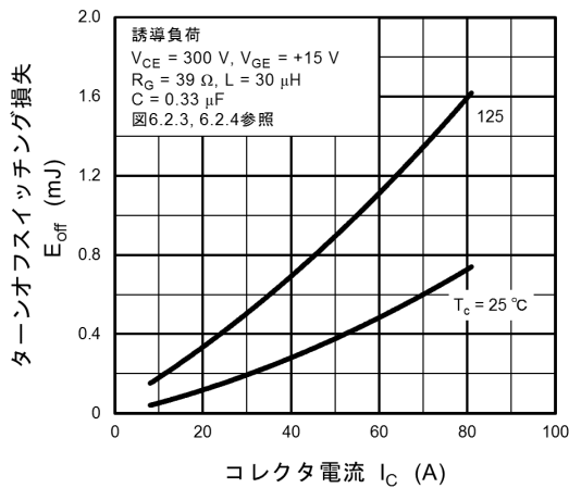
図 8.15 E_{\text{off}} - I_C
