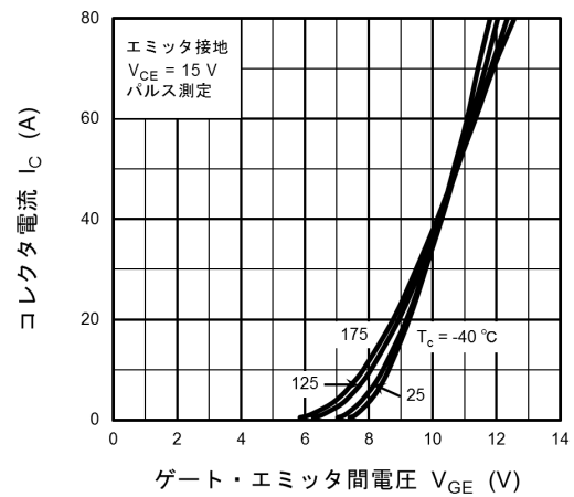
図 8.6 I_c - V_{GE}
