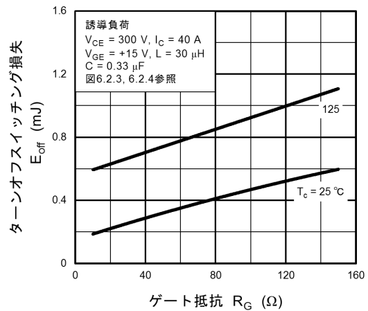
図 8.16 E_{\text{off}} - R_G
