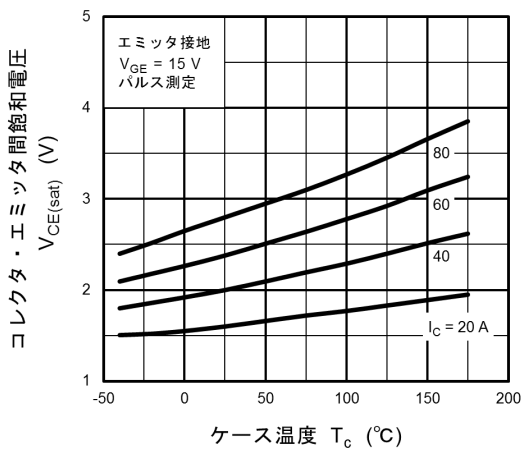
図 8.5 V_{CE(sat)} - T_c
