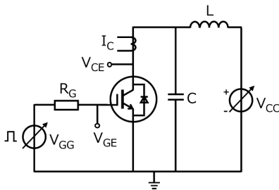
図 6.2.1 スwitchング時間の測定回路
