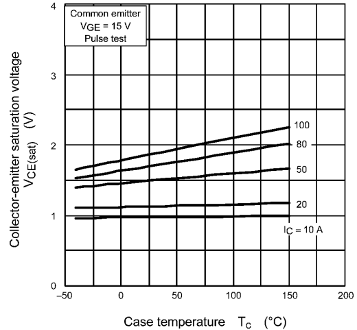
Fig. 8.4 V_{CE(sat)} - T_c
