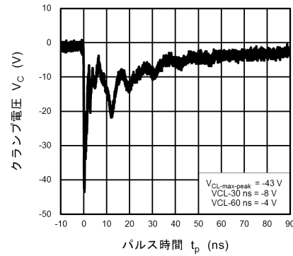
図 10.19.4 IEC61000-4-2 クランプ波形 -8 kV
