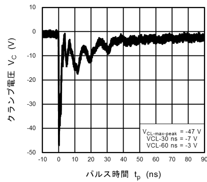
図 10.20.4 IEC61000-4-2 クランプ波形 -8 kV
