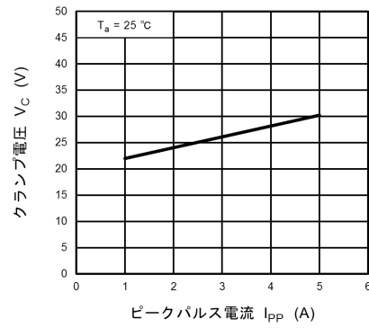
図 10.15.2 V_C - I_{PP}
