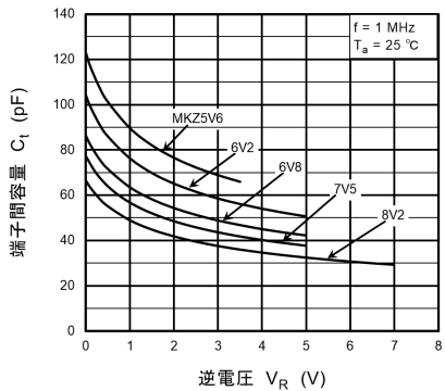
図 10.1.5 C_t - V_R(1)
