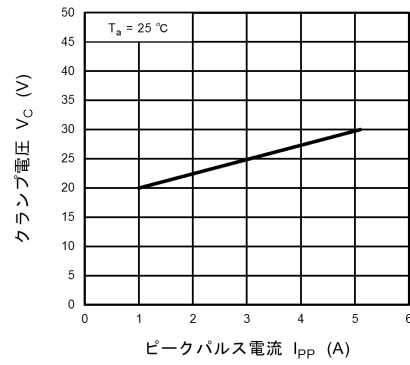
図 10.14.2 V_C - I_{PP}
