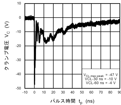
図 10.9.4 IEC61000-4-2 クランプ波形 -8 kV
