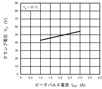
図 10.21.2 V_C - I_{PP}
