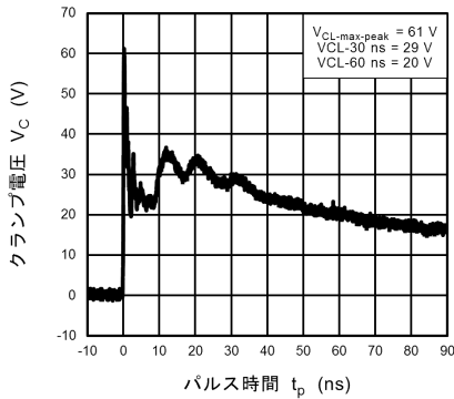
図 10.10.3 IEC61000-4-2 クランプ波形 +8 kV
