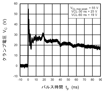
図 10.12.3 IEC61000-4-2 クランプ波形 +8 kV
