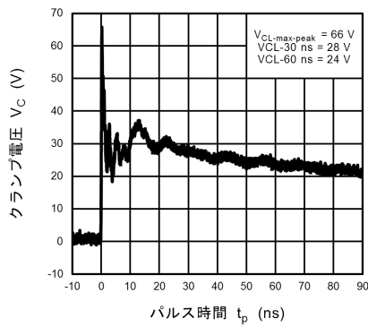
図 10.14.3 IEC61000-4-2 クランプ波形 +8 kV
