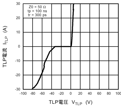
図 10.20.1 I_{TLP} - V_{TLP}
