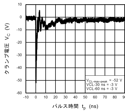
図 10.14.4 IEC61000-4-2 クランプ波形 -8 kV
