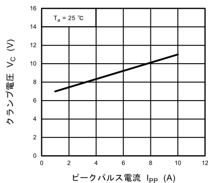
図 10.4.2 V_C - I_{PP}
