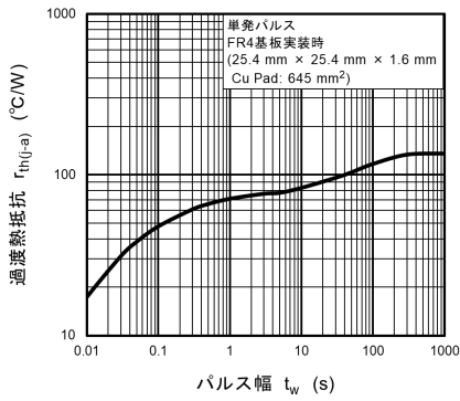
図 10.1.11 r_{th(j-a)} - t_w
