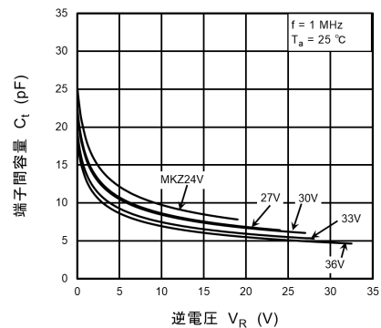
図 10.1.8 C_t - V_R(4)
