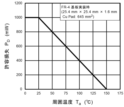
図 10.1.10 P_D - T_a
