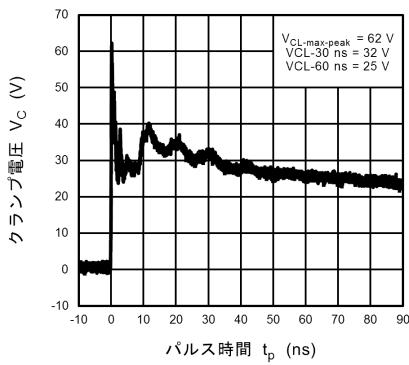
図 10.15.3 IEC61000-4-2 クランプ波形 +8 kV
