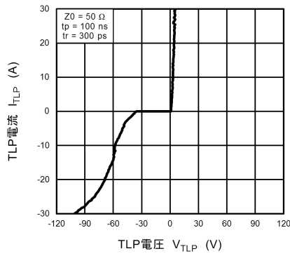
図 10.21.1 I_{TLP} - V_{TLP}
