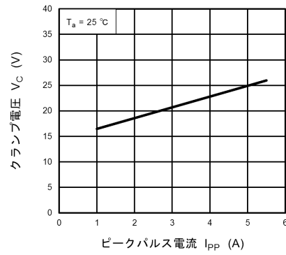
図 10.13.2 V_C - I_{PP}
