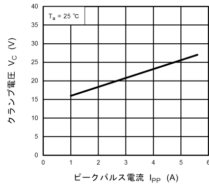
図 10.12.2 V_C - I_{PP}
