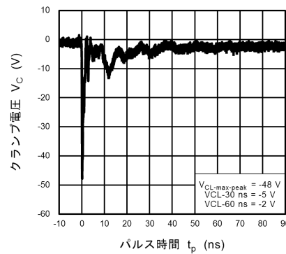
図 10.16.4 IEC61000-4-2 クランプ波形 -8 kV
