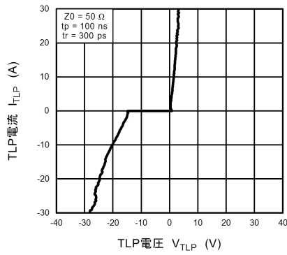
図 10.12.1 I_{TLP} - V_{TLP}
