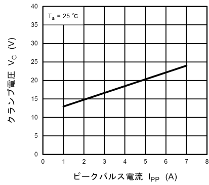
図 10.10.2 V_C - I_{PP}
