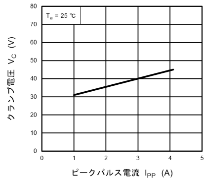
図 10.18.2 V_C - I_{PP}
