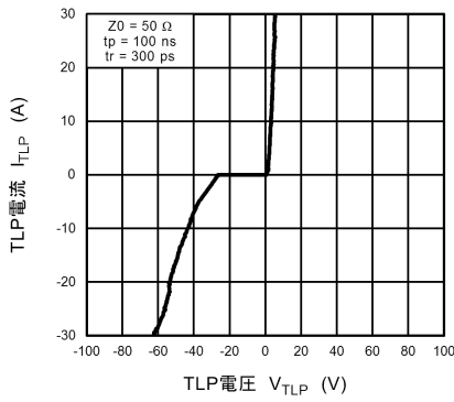
図 10.18.1 I_{TLP} - V_{TLP}
