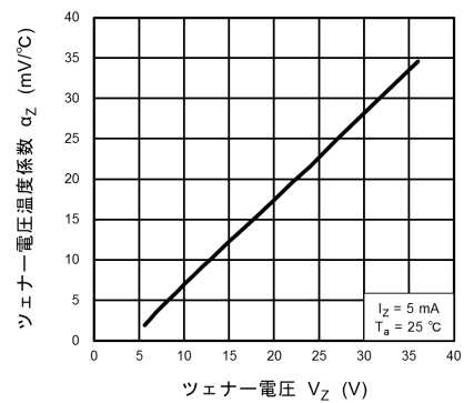
図 10.1.4 \alpha_Z - V_Z
