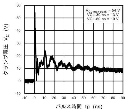
図 10.4.3 IEC61000-4-2 クランプ波形 +8 kV
