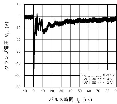
図 10.15.4 IEC61000-4-2 クランプ波形 -8 kV
