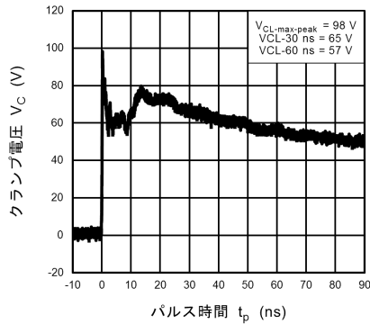
図 10.21.3 IEC61000-4-2 クランプ波形 +8 kV
