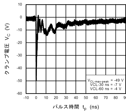
図 10.17.4 IEC61000-4-2 クランプ波形 -8 kV
