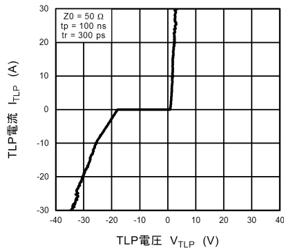
図 10.14.1 I_{TLP} - V_{TLP}
