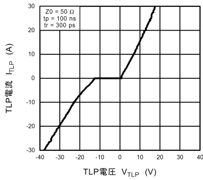
図 10.11.1 I_{TLP} - V_{TLP}
