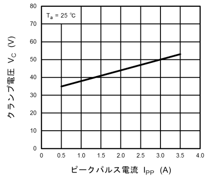
図 10.20.2 V_C - I_{PP}
