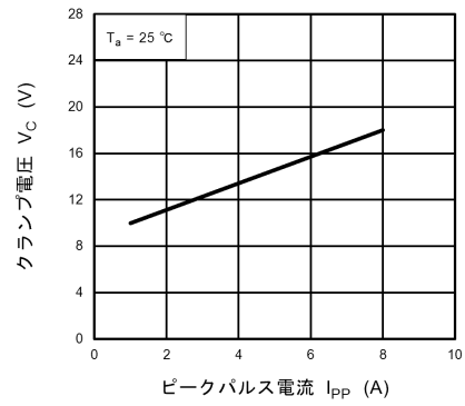
図 10.7.2 V_C - I_{PP}
