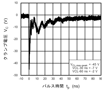
図 10.18.4 IEC61000-4-2 クランプ波形 -8 kV
