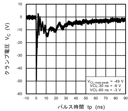
図 10.6.4 IEC61000-4-2 クランプ波形 -8 kV
