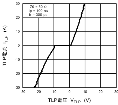
図 10.8.1 I_{TLP} - V_{TLP}
