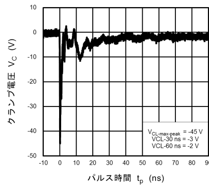
図 10.12.4 IEC61000-4-2 クランプ波形 -8 kV
