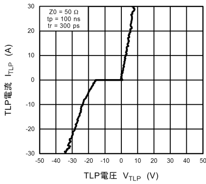
図 10.13.1 I_{TLP} - V_{TLP}
