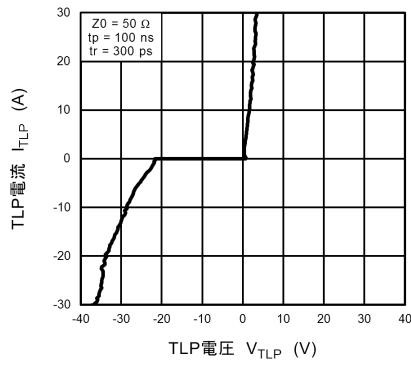
図 10.16.1 I_{TLP} - V_{TLP}
