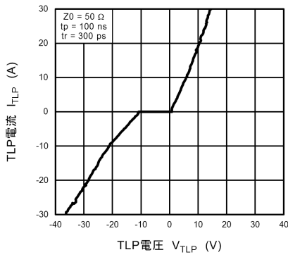
図 10.9.1 I_{TLP} - V_{TLP}
