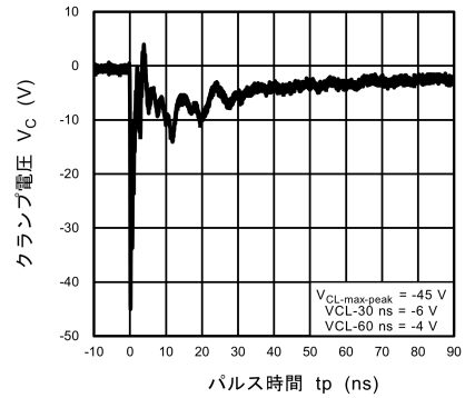
図 10.5.4 IEC61000-4-2 クランプ波形 -8 kV
