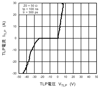
図 10.17.1 I_{TLP} - V_{TLP}
