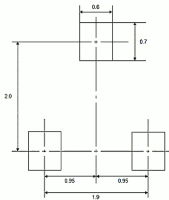
図 9.1 参考パッド寸法(Unit: mm)
