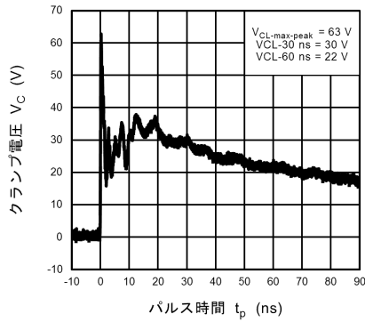
図 10.11.3 IEC61000-4-2 クランプ波形 +8 kV
