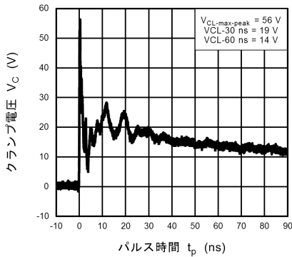
図 10.8.3 IEC61000-4-2 クランプ波形 +8 kV
