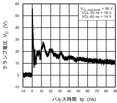
図 10.6.3 IEC61000-4-2 クランプ波形 +8 kV
