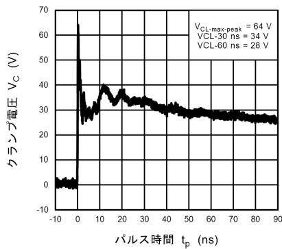
図 10.16.3 IEC61000-4-2 クランプ波形 +8 kV
