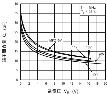
図 10.1.7 C_t - V_R(3)
