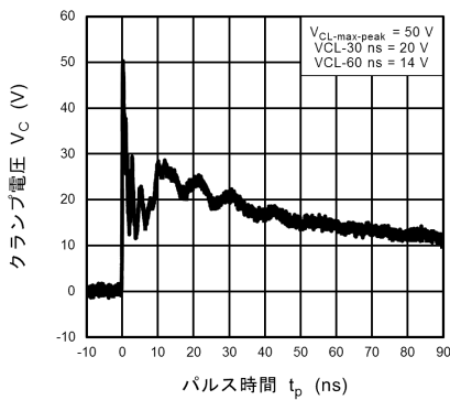
図 10.7.3 IEC61000-4-2 クランプ波形 +8 kV
