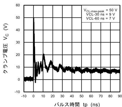
図 10.2.3 IEC61000-4-2 クランプ波形 +8 kV
