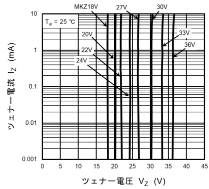
図 10.1.2 I_Z - V_Z(2)
