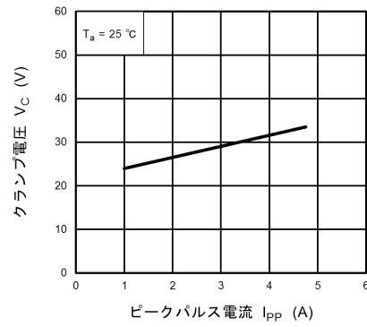
図 10.16.2 V_C - I_{PP}
