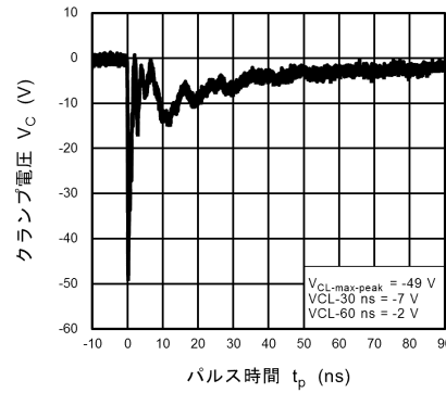
図 10.13.4 IEC61000-4-2 クランプ波形 -8 kV
