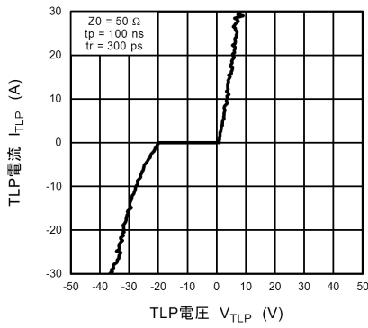
図 10.15.1 I_{TLP} - V_{TLP}
