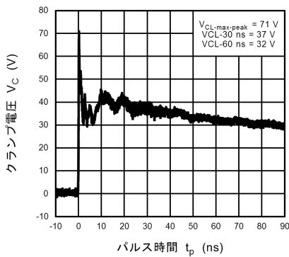
図 10.17.3 IEC61000-4-2 クランプ波形 +8 kV
