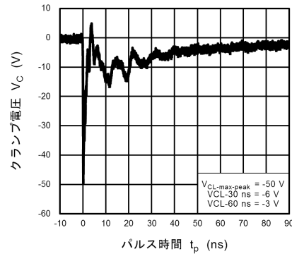
図 10.8.4 IEC61000-4-2 クランプ波形 -8 kV
