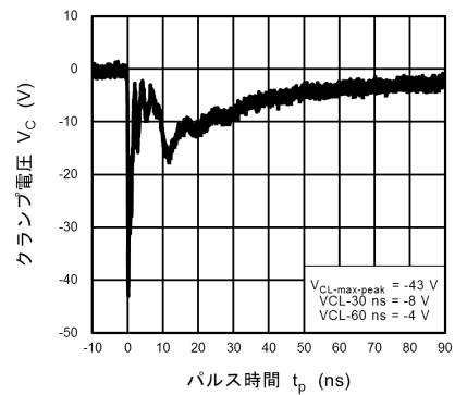
図 10.7.4 IEC61000-4-2 クランプ波形 -8 kV
