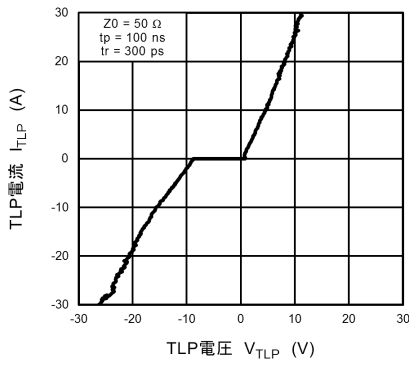
図 10.7.1 I_{TLP} - V_{TLP}
