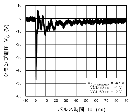
図 10.2.4 IEC61000-4-2 クランプ波形 -8 kV
