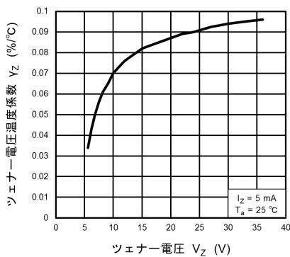
図 10.1.3 \gamma_Z - V_Z
