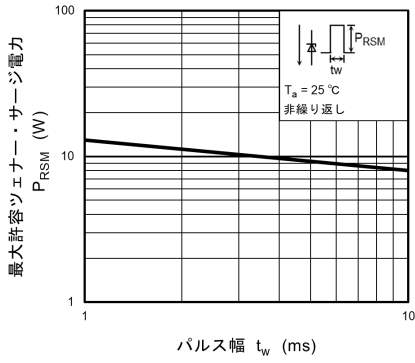
図 10.1.9 P_{RSM} - t_w
