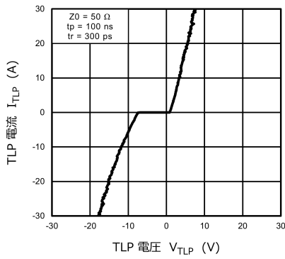
図 10.5.1 I_{TLP} - V_{TLP}
