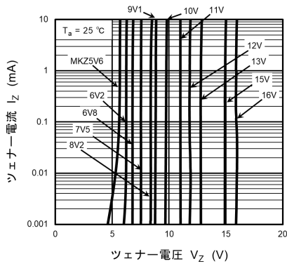
図 10.1.1 I_Z - V_Z(1)
