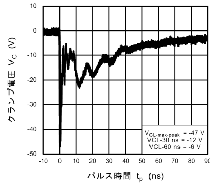
図 10.11.4 IEC61000-4-2 クランプ波形 -8 kV
