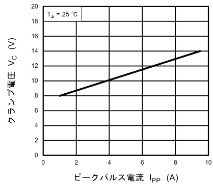
図 10.5.2 V_C - I_{PP}
