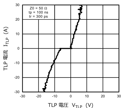
図 10.4.1 I_{TLP} - V_{TLP}
