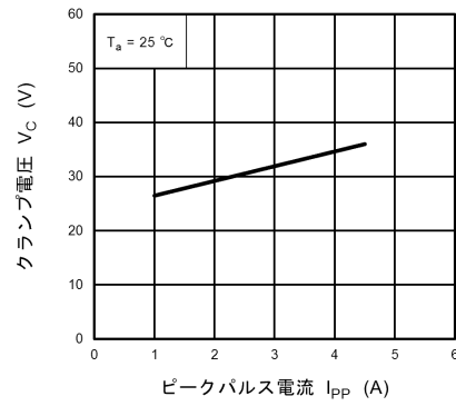
図 10.17.2 V_C - I_{PP}
