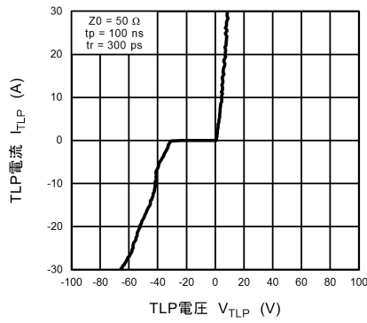
図 10.19.1 I_{TLP} - V_{TLP}
