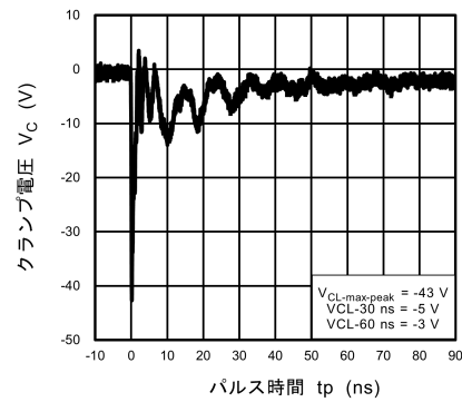
図 10.3.4 IEC61000-4-2 クランプ波形 -8 kV
