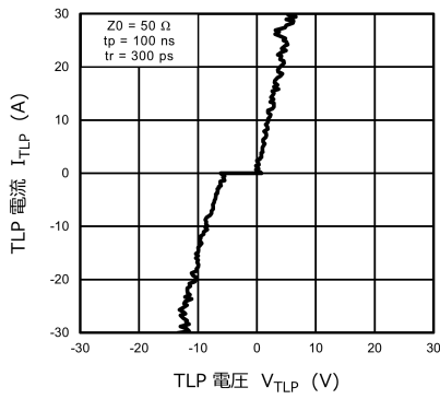
図 10.3.1 I_{TLP} - V_{TLP}
