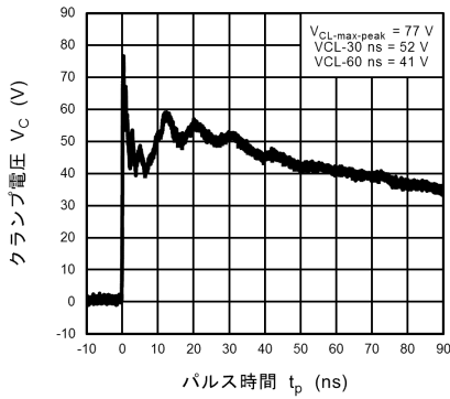
図 10.18.3 IEC61000-4-2 クランプ波形 +8 kV
