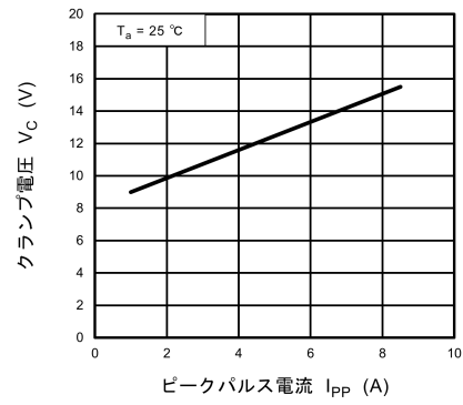
図 10.6.2 V_C - I_{PP}
