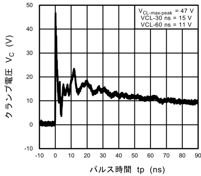
図 10.5.3 IEC61000-4-2 クランプ波形 +8 kV
