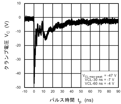
図 10.21.4 IEC61000-4-2 クランプ波形 -8 kV
