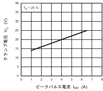
図 10.11.2 V_C - I_{PP}
