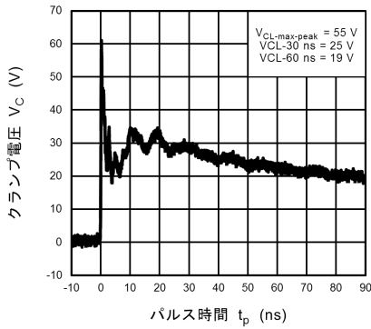
図 10.13.3 IEC61000-4-2 クランプ波形 +8 kV
