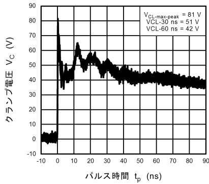
図 10.19.3 IEC61000-4-2 クランプ波形 +8 kV
