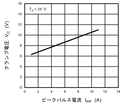
図 10.3.2 V_C - I_{PP}
