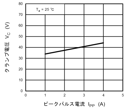
図 10.19.2 V_C - I_{PP}
