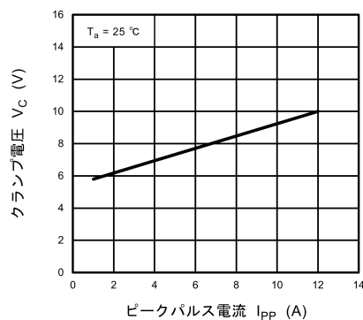
図 10.2.2 V_C - I_{PP}
