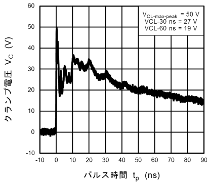
図 10.9.3 IEC61000-4-2 クランプ波形 +8 kV
