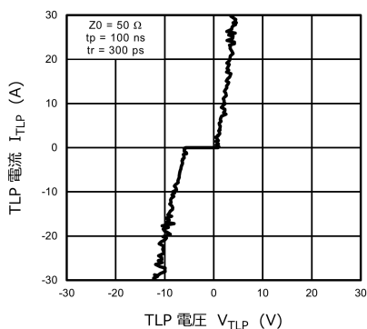
図 10.2.1 I_{TLP} - V_{TLP}
