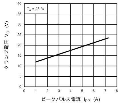
図 10.9.2 V_C - I_{PP}
