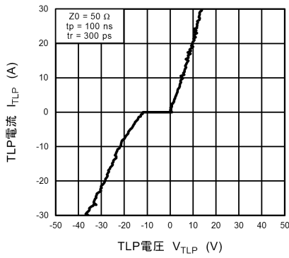
図 10.10.1 I_{TLP} - V_{TLP}
