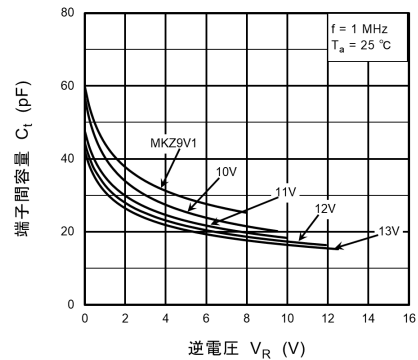
図 10.1.6 C_t - V_R(2)
