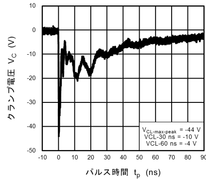
図 10.10.4 IEC61000-4-2 クランプ波形 -8 kV
