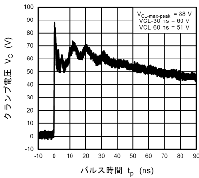
図 10.20.3 IEC61000-4-2 クランプ波形 +8 kV
