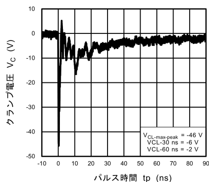
図 10.4.4 IEC61000-4-2 クランプ波形 -8 kV
