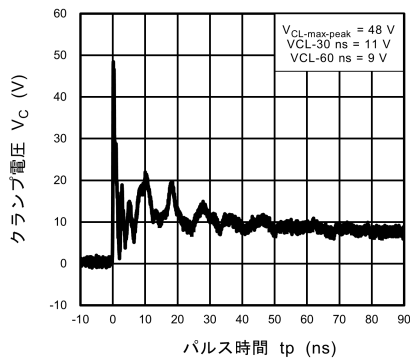
図 10.3.3 IEC61000-4-2 クランプ波形 +8 kV
