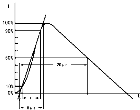
図 10.22.1 V_C - I_{PP} 印加波形 (IEC61000-4-5準拠 8/20μs pulse)
