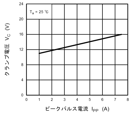
図 10.8.2 V_C - I_{PP}
