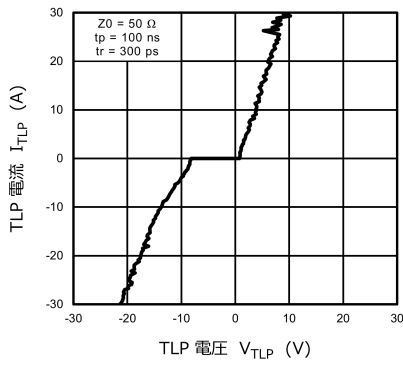
図 10.6.1 I_{TLP} - V_{TLP}
