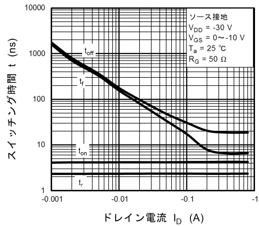
図 8.10 t - I_D
