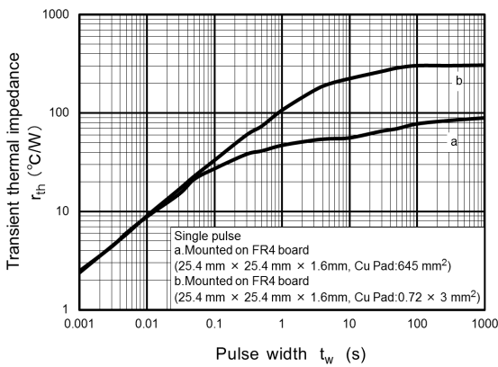
Fig. 7.11 r_{th} - t_w
