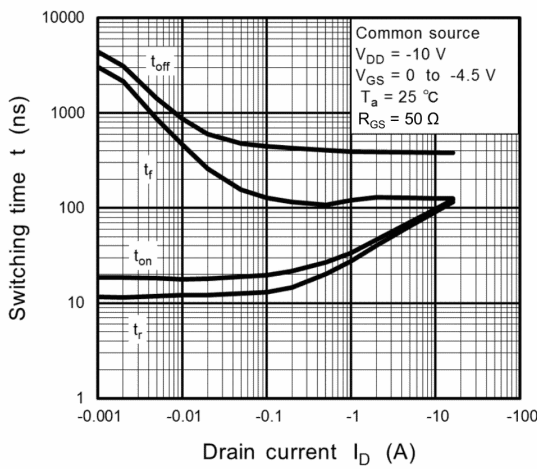
Fig. 7.9 t - I_D
