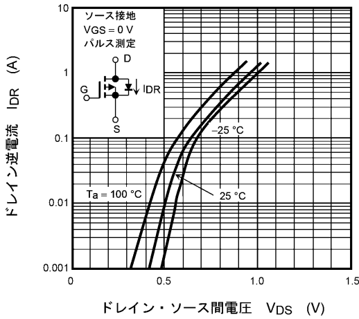
図 8.9 I_{DR} - V_{DS}
