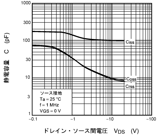
図 8.10 C - V_{DS}
