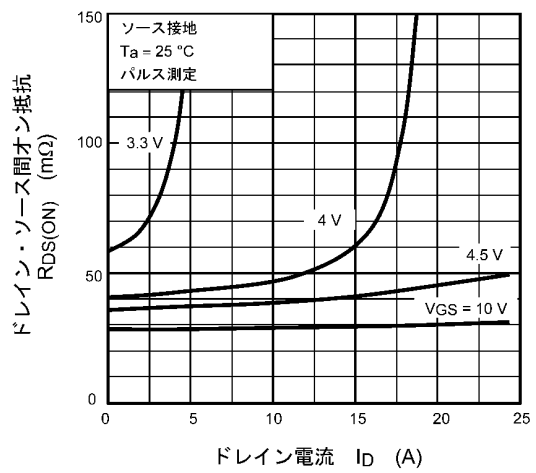
図 8.4 R_{DS(ON)} - I_D
