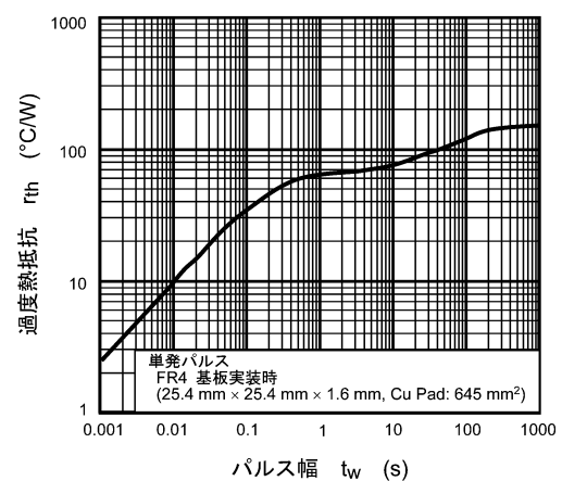
図 8.12 rth - tw
