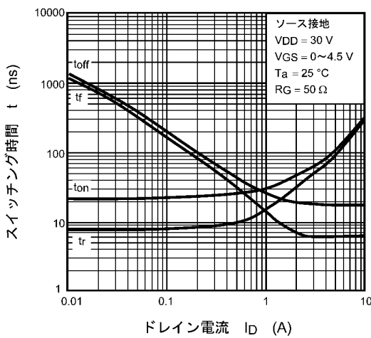
図 8.9 t - ID
