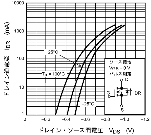
図 7.8 I_{DR} - V_{DS}
