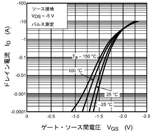
図 8.2 I_D - V_{GS}
