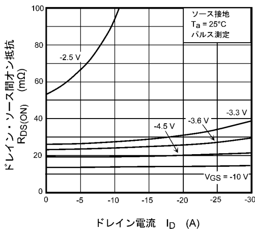
図 8.5 R_{DS(ON)} - I_D
