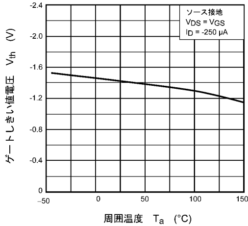
図 8.7 V_{th} - T_a
