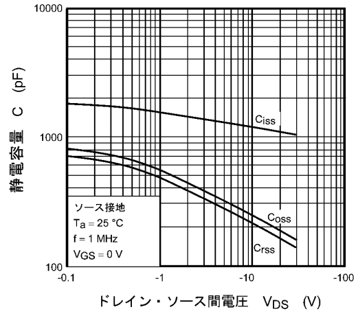
図 8.8 C - V_{DS}
