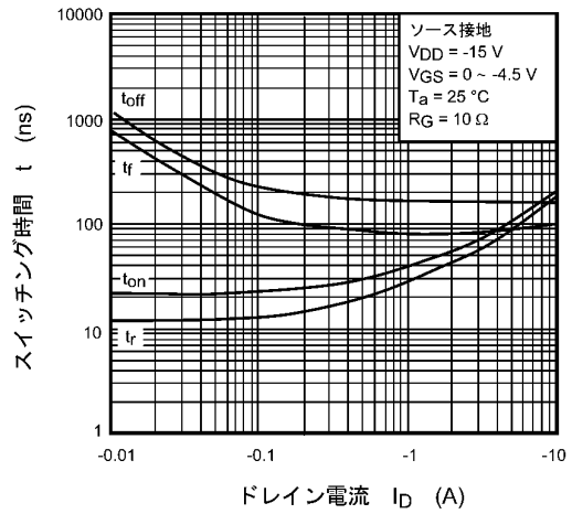
図 8.10 t - I_D
