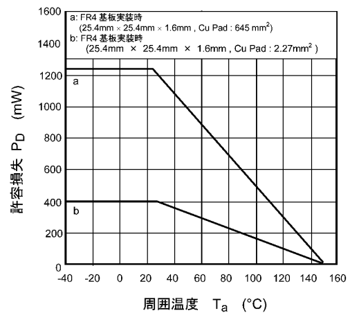
図 8.12 P_D - T_a
