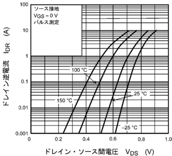
図 8.11 I_{DR} - V_{DS}
