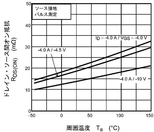
図 8.6 R_{DS(ON)} - T_a
