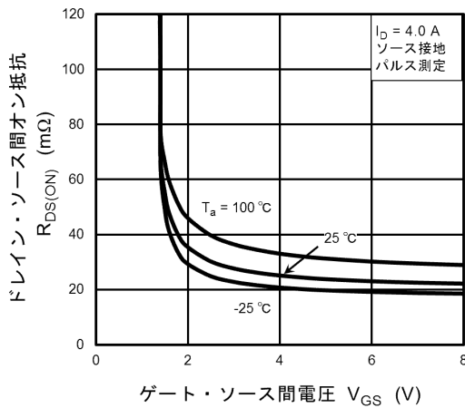
図 8.3 R_{DS(ON)} - V_{GS}
