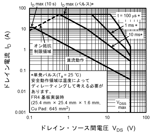
図 7.14 安全動作領域
