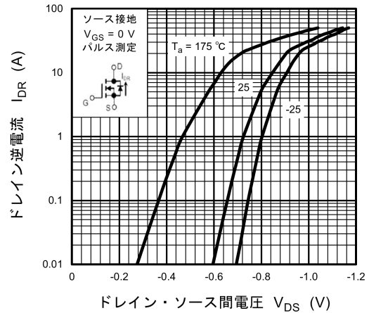
図 7.8 I_{DR} - V_{DS}
