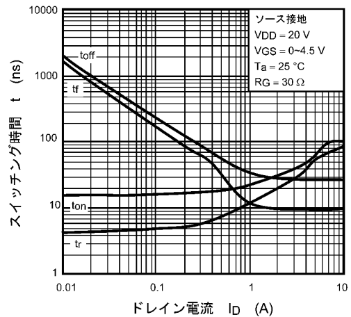
図 7.10 t - I_D
