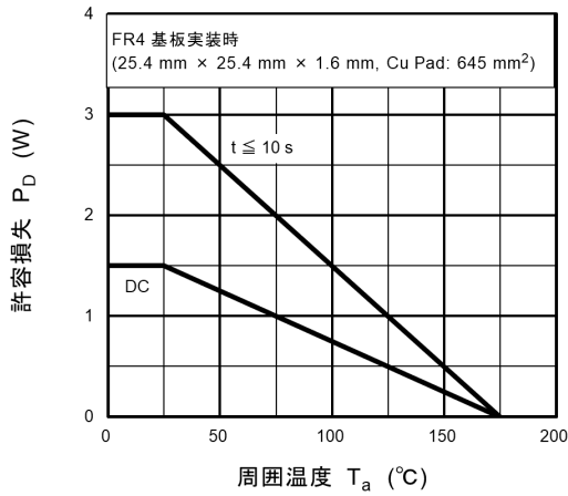
図 7.13 P_D - T_a
