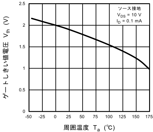
図 7.7 V_{th} - T_a
