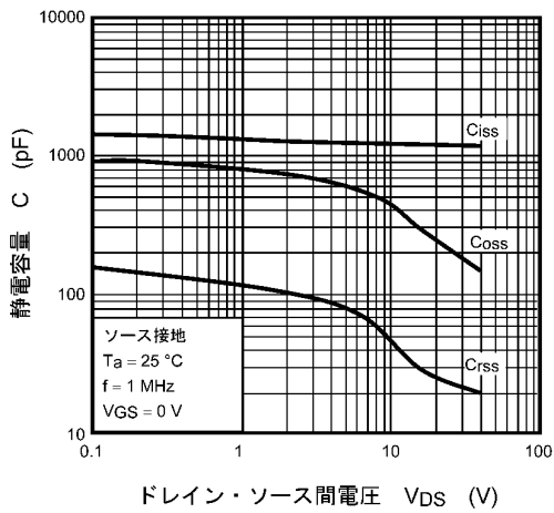
図 7.9 C - V_{DS}
