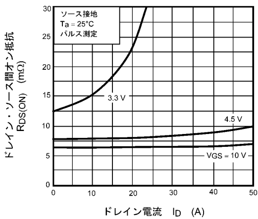
図 7.5 R_{DS(ON)} - I_D
