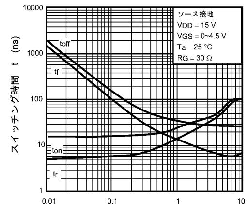
図 7.10 t - I_D
