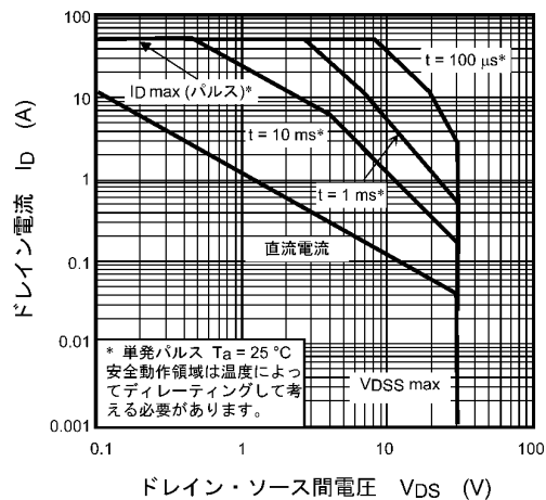
図 7.14 安全動作領域
