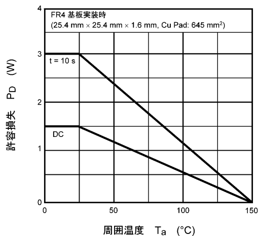
図 7.13 P_D - T_a
