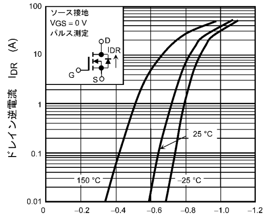
図 7.8 I_{DR} - V_{DS}
