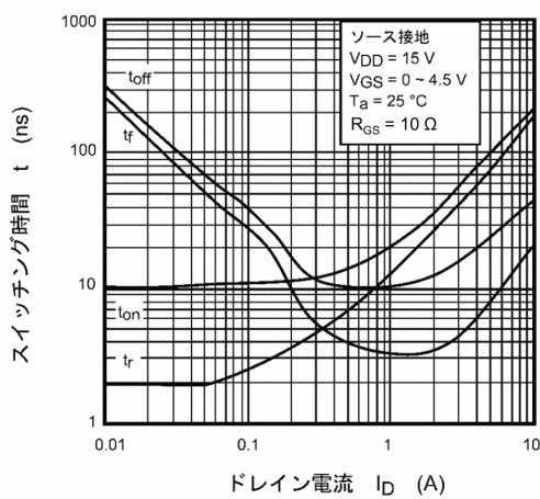
図 8.11 t - I_D
