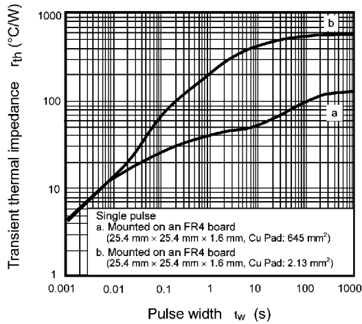
図 8.13 r_{th} - t_w
