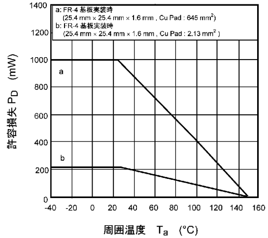
図 8.14 P_D - T_a
