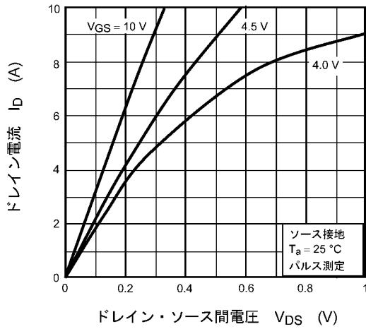
図 8.1 I_D - V_{DS}
