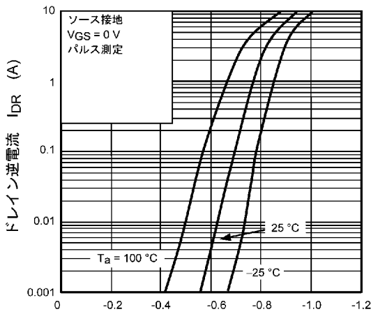
図 8.9 I_{DR} - V_{DS}
