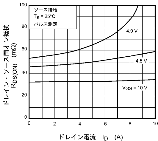
図 8.5 R_{DS(ON)} - I_D
