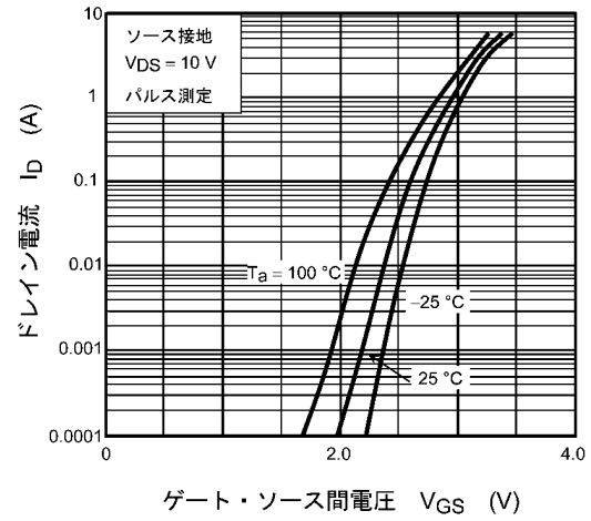
図 8.2 I_D - V_{GS}
