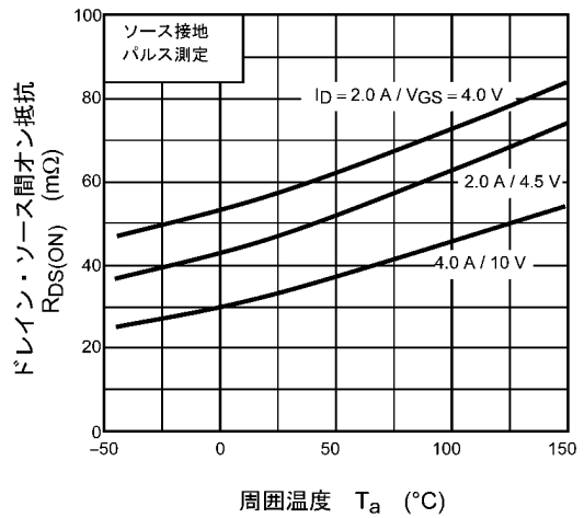
図 8.6 R_{DS(ON)} - T_a
