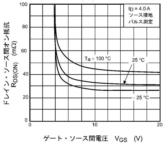
図 8.4 R_{DS(ON)} - V_{GS}
