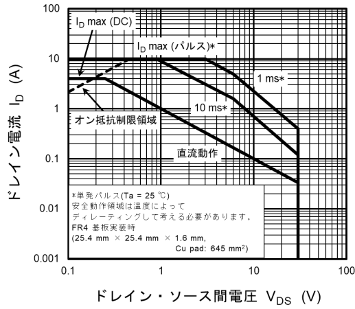
図 8.15 安全動作領域
