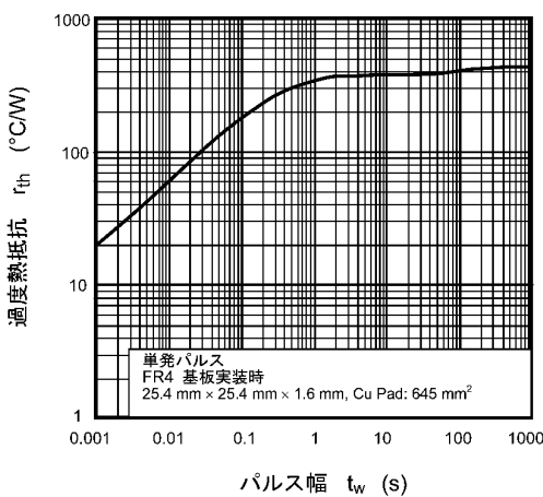
図 8.11 r_{th} - t_w
