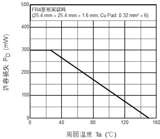
図 7.11 P_D - T_a
