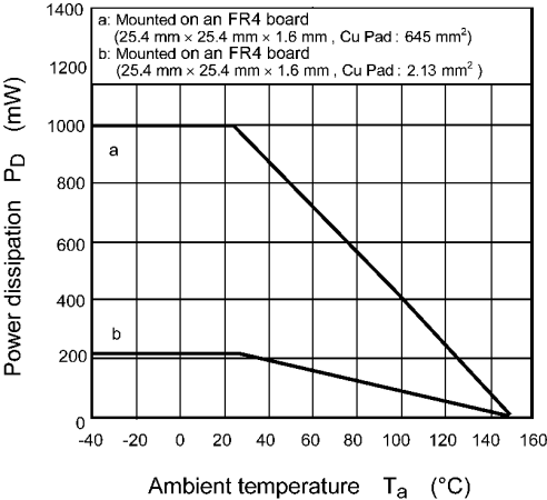
Fig. 9.13 P_D - T_a
