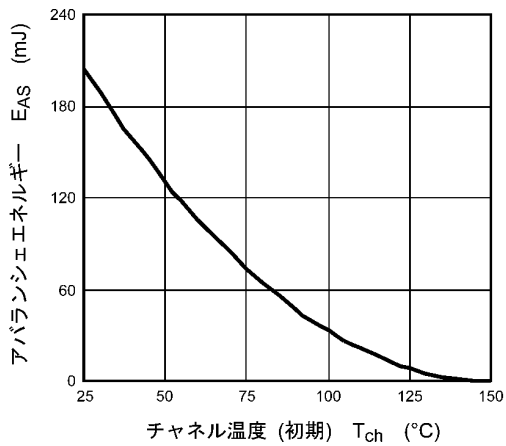
アバランジエエエネルギー E_{AS} (mJ) チャネル温度 (初期) T_{ch} (°C) 図 8.14 E_{AS} - T_{ch} (最大値 (保証値))
