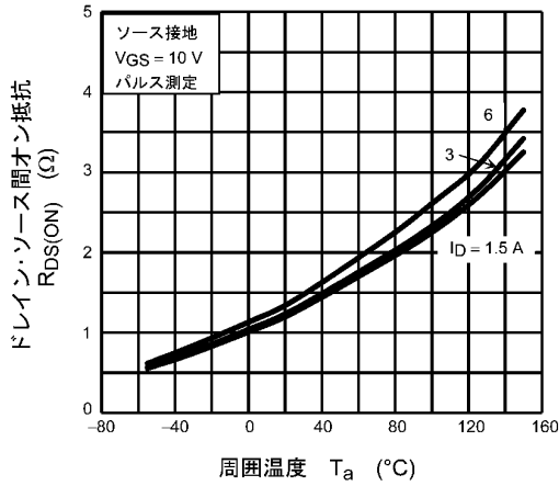
図 8.7 R_{DS(ON)} - T_a
