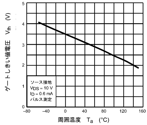
図 8.10 V_{th} - T_a
