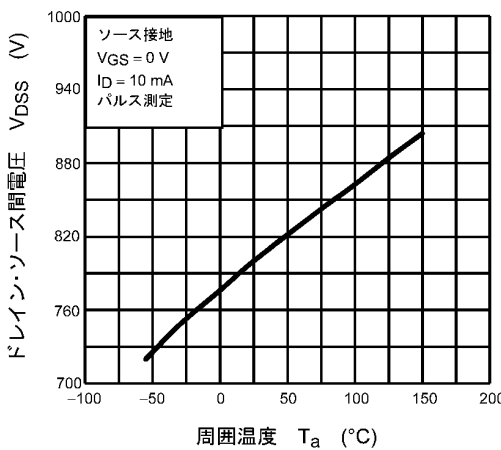
図 8.5 V_{DS} - T_a
