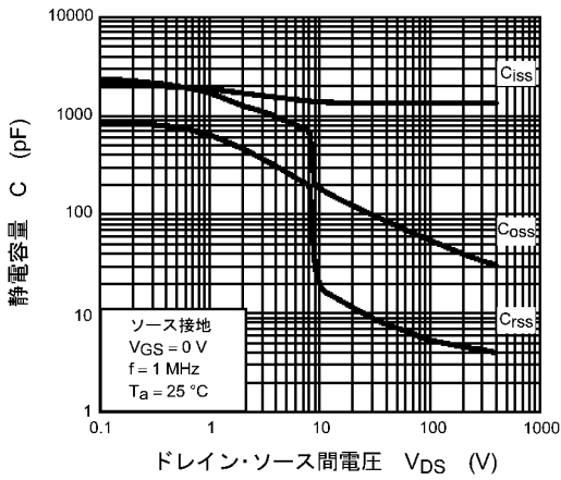
図 8.9 C - V_{DS}
