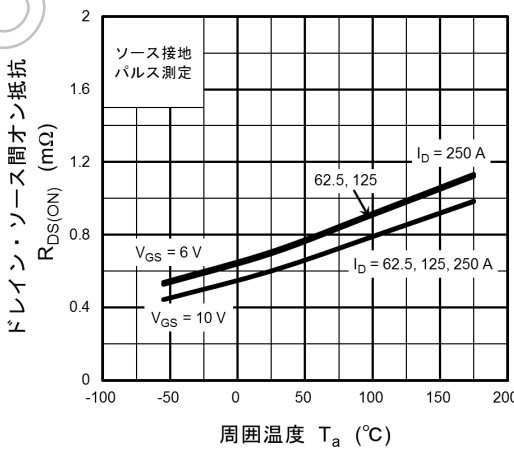
図 9.6 R_{DS(ON)} - T_a
