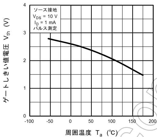
図 9.9 V_{th} - T_a
