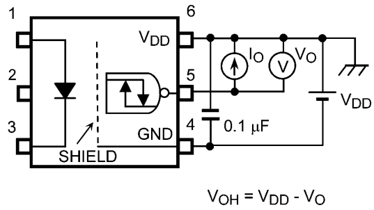
図 12.1.2 VOH測定回路
