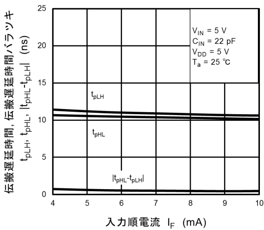
図 12.2.15 t_{pHL} , t_{pLH} , |t_{pHL} - t_{pLH}| - I_F
